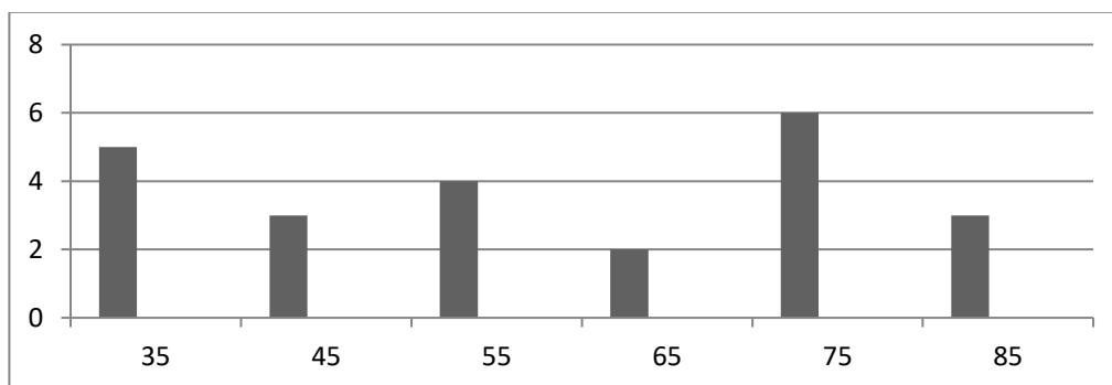
Gambar 3 Histogram Kelas Kontrol
