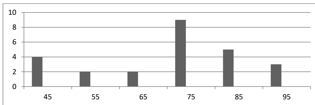
Gambar 2 Histogram Kelas Ekperimen
