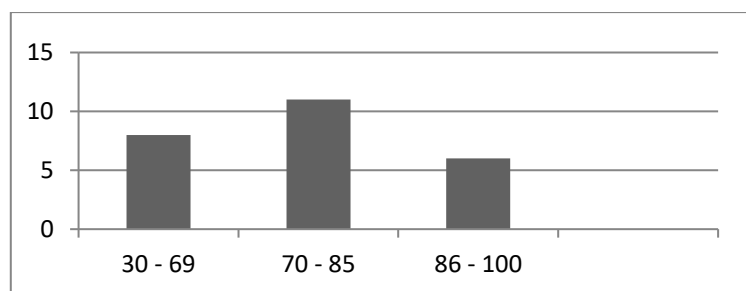
Gambar 1 Histogram Kelas Eksperimen Ujian Tengah Semester
