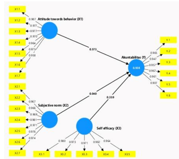
Gambar 1. Model Persamaan Struktural
