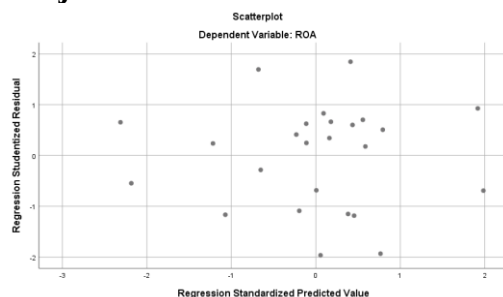
Gambar 2. Uji Heteroksistas Sumber : data diolah, 2021
