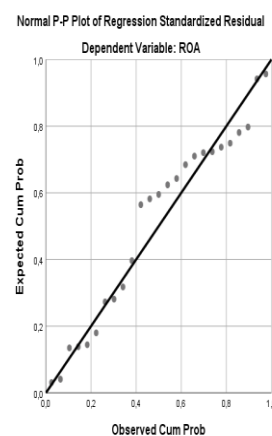
Gambar 3. Uji Normalitas Sumber : data diolah, 2021
