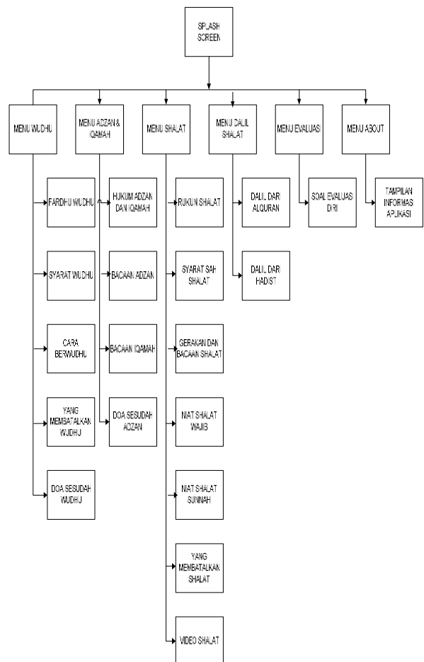
Gambar 6. Struktur Program
