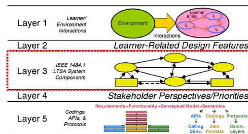
Gambar 1. Arsitektur LTSA
