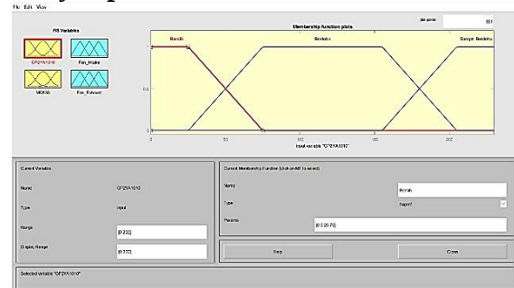
Gambar 3. Fungsi Keanggotaan Input GP2Y1010AU0F
