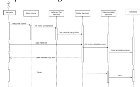
Gambar 16. Sequence Diagram Pemesanan
