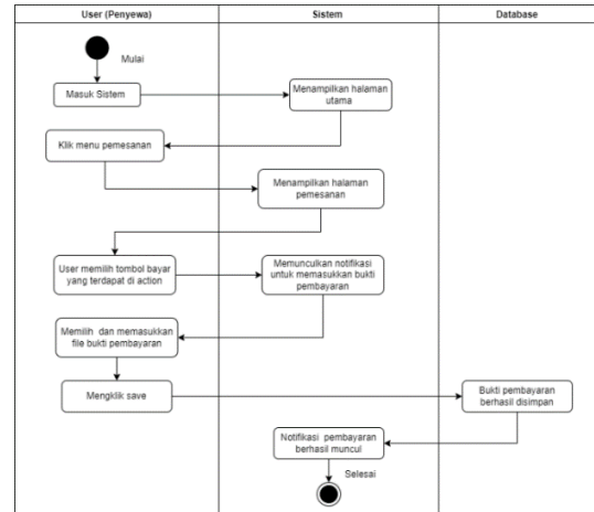
Gambar 7. Activity Diagram Pembayaran
