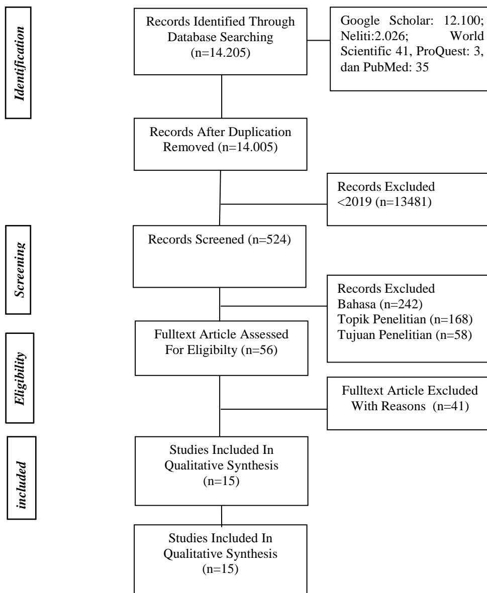
Gambar. 1 Algoritma Pencarian
